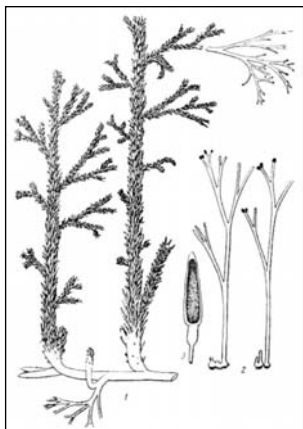
Древнейшие растения суши псилофиты
