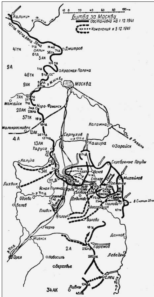
Схема боев на подступах к Кашире из книги воспоминаний Гудериана
