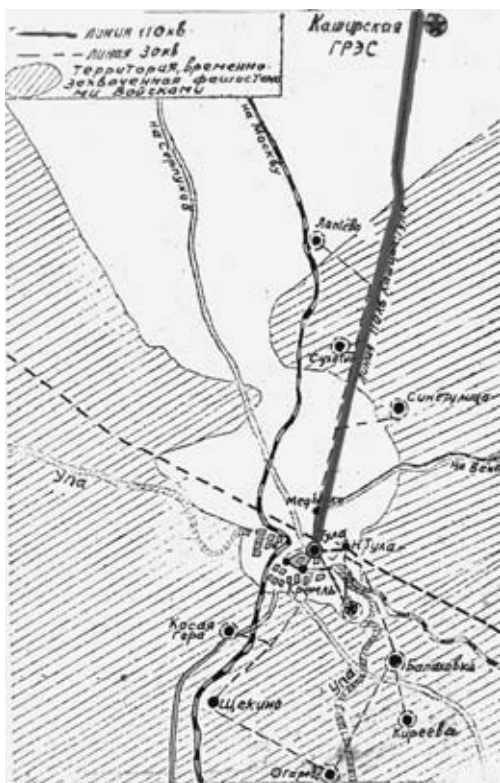
Схема прохождения линия электропередачи по которой из Каширы в осажденную Тулу поступала электроэнергия
